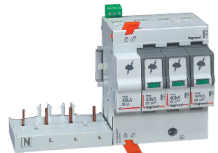
УЗИП типа T2, стыкуемые с автоматическим выключателем
